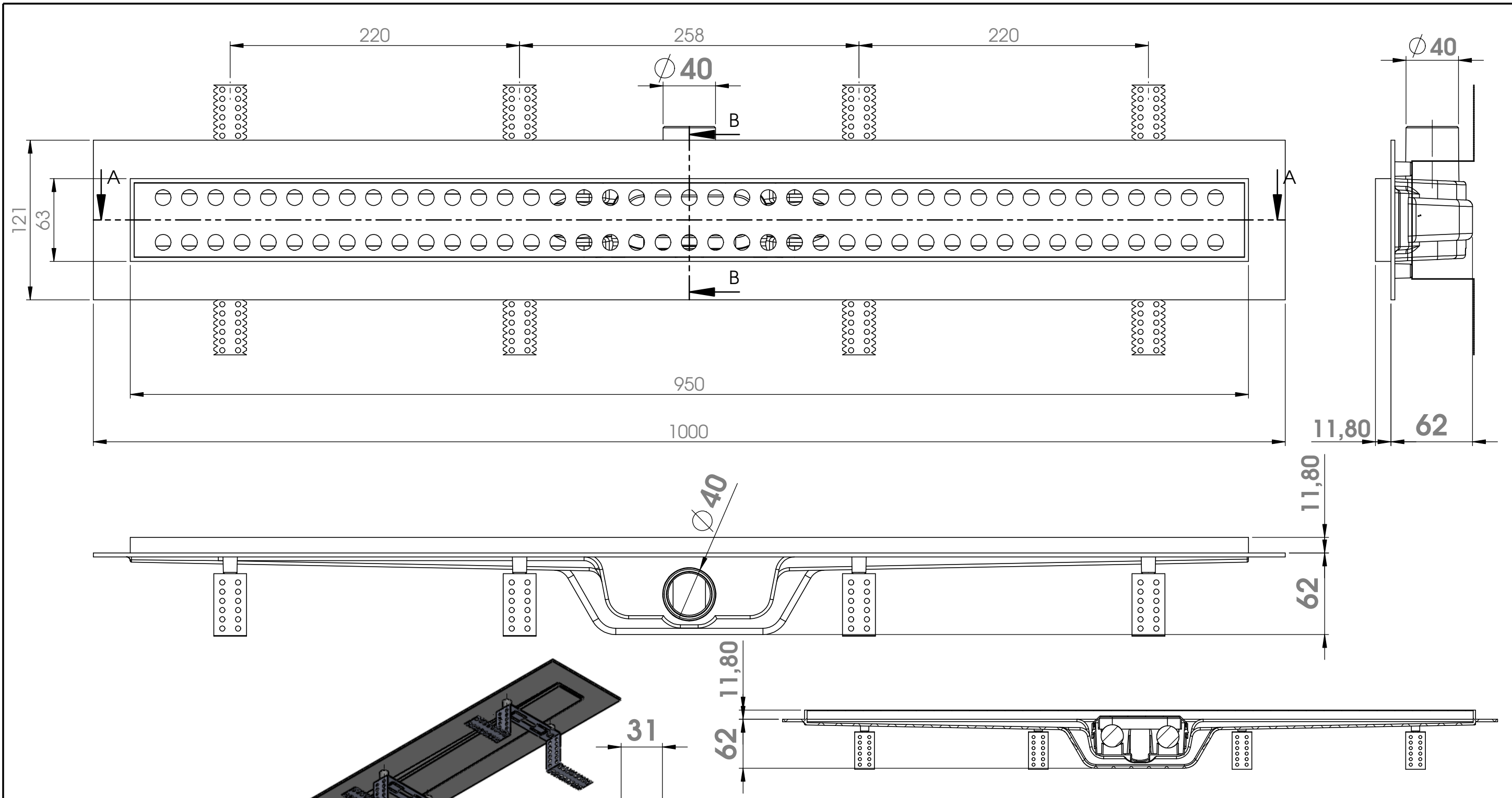
SECTION A-A
